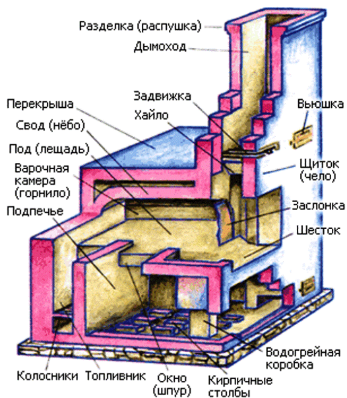
Устройство русской печи
