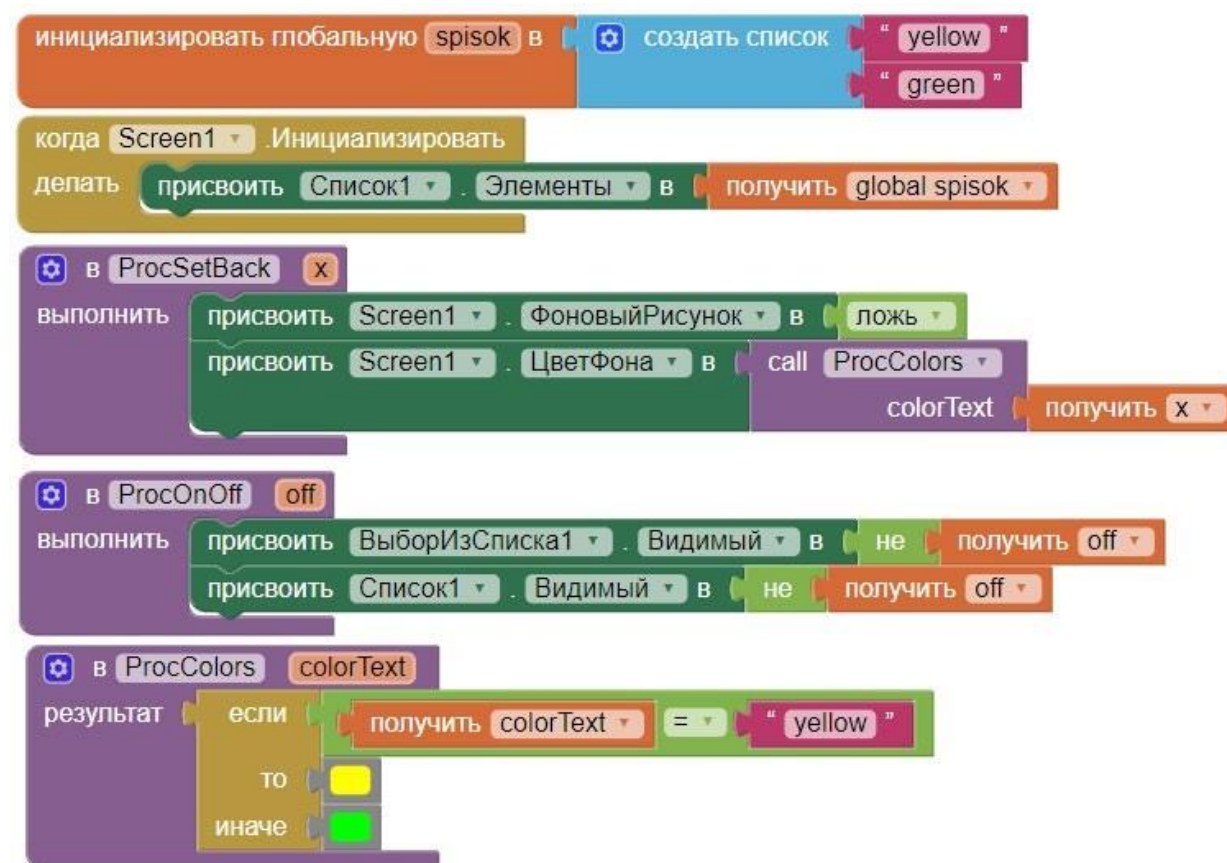
Рисунок 177. Финальный вид схемы блоков приложения, часть 1
