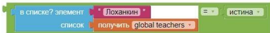
Рисунок 138. Логическое выражение с блоком проверки
