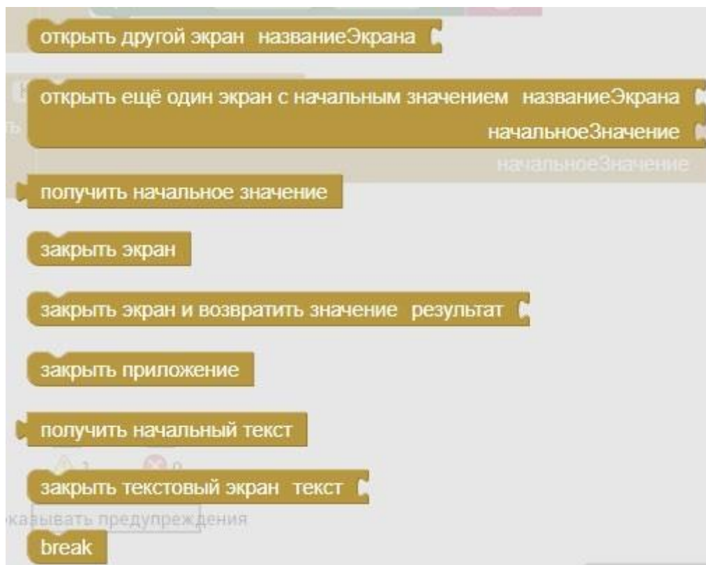
Рисунок 228. Блоки управления экранами
