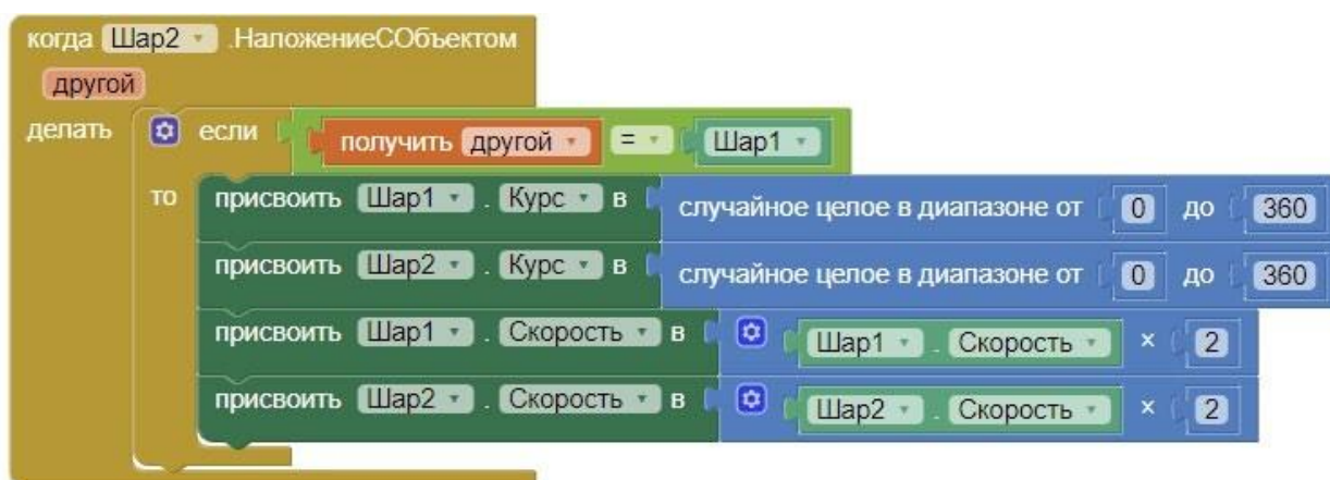
Рисунок 213. Обработчик столкновений шаров друг с другом
