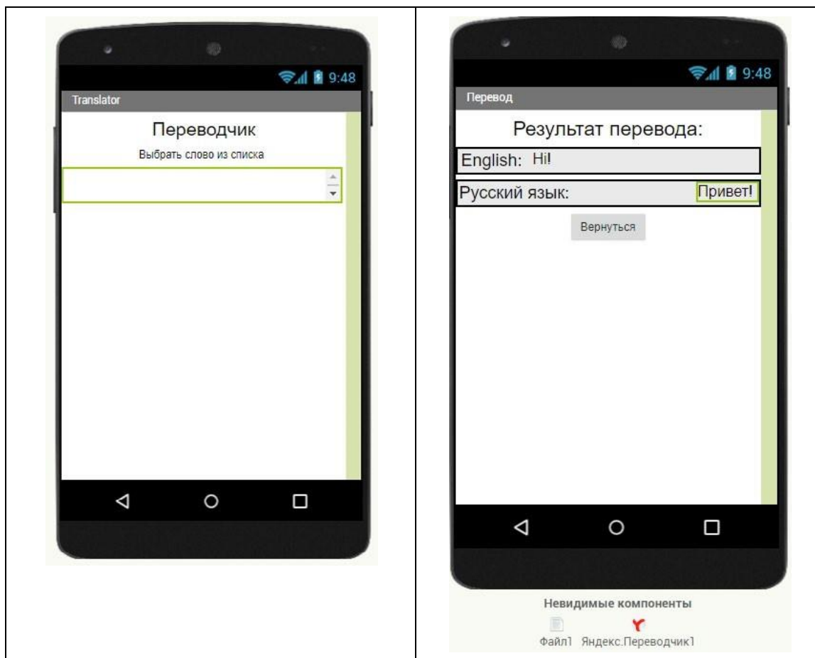
Рисунок 233. Примерная схема дизайна экранов приложения
