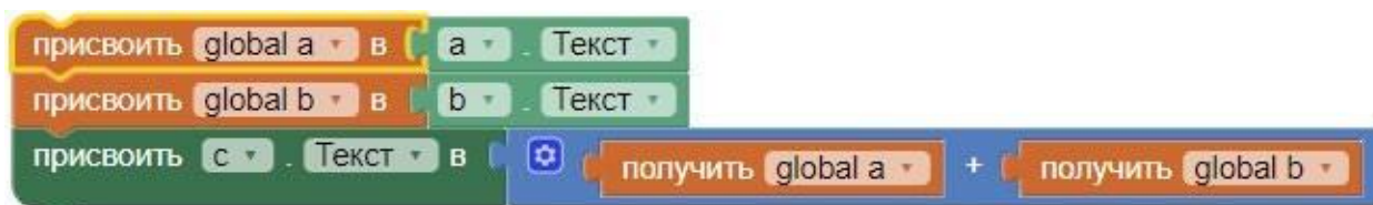
Рисунок 127. Итоговый вид блоков обработчика кнопки операции сложения
