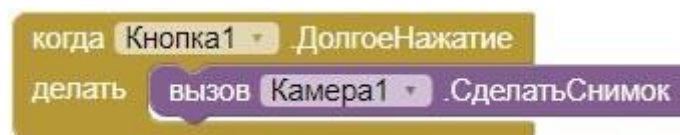
Рисунок 287. Обработчик события «долгое нажатие» на кнопку
