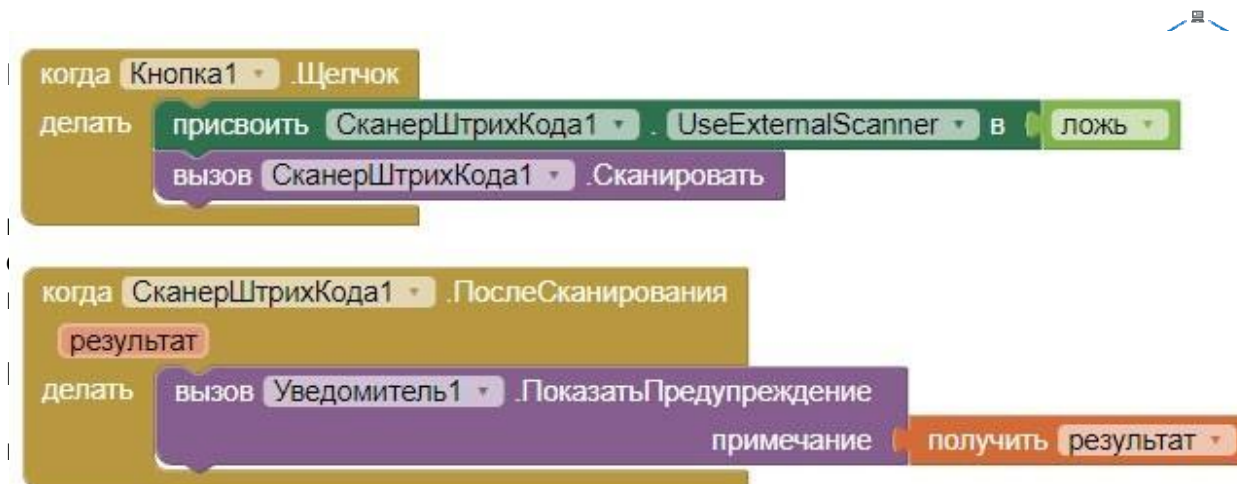
Рисунок 308. Блоки для работы с компонентой СканерШтрихКода1
