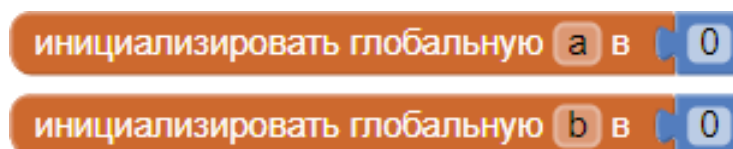
Рисунок 123. Инициализация переменных
