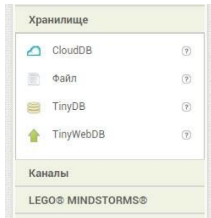
Рисунок 43. Функционал «Хранилище»
