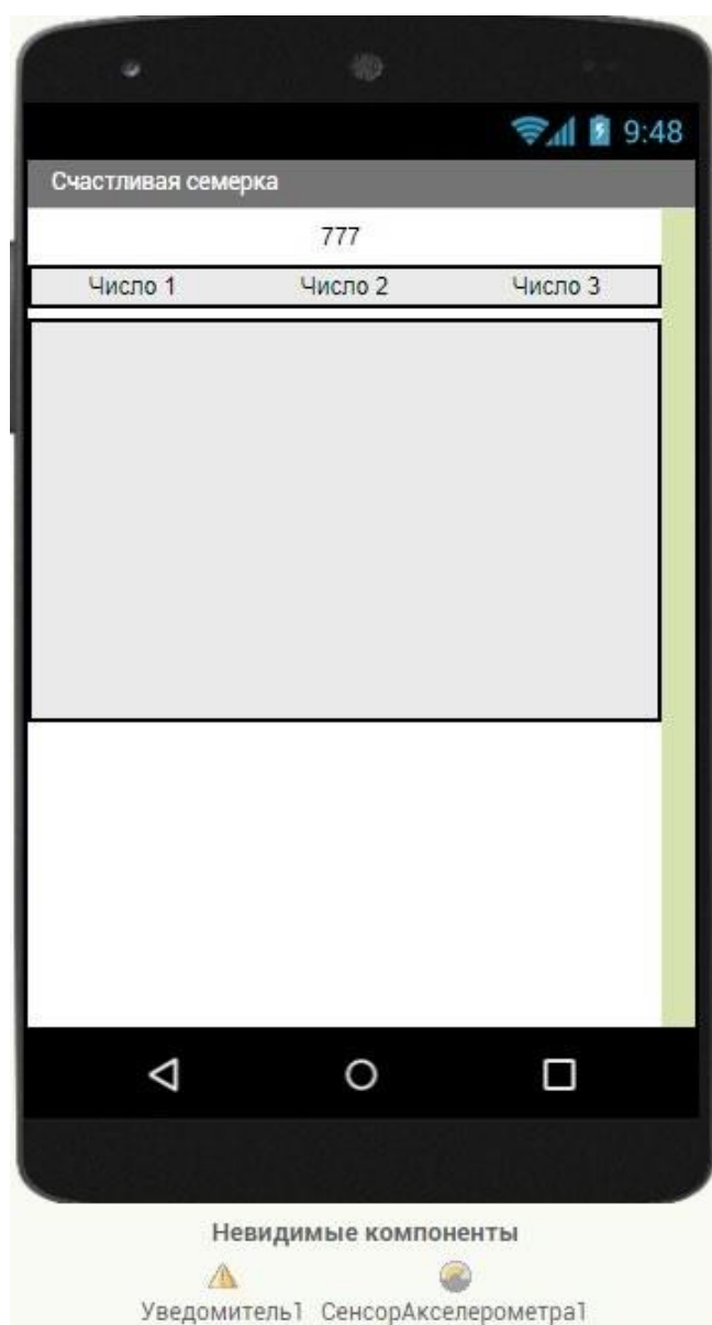
Рисунок 183. Дизайн приложения
