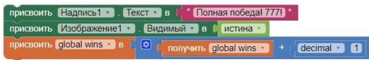
Рисунок 196. Сеттеры для компонент Надпись1, Изображение1 и переменной wins в случае выигрыша
