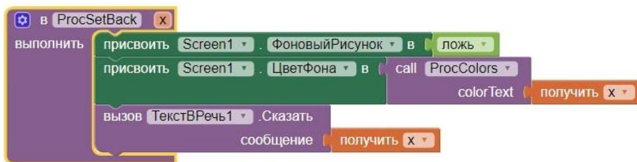
Рисунок 179. Модификация процедуры ProcSetBack
