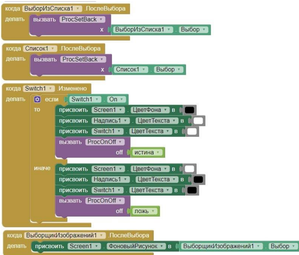
Рисунок 178. Финальный вид схемы блоков приложения, часть 2
