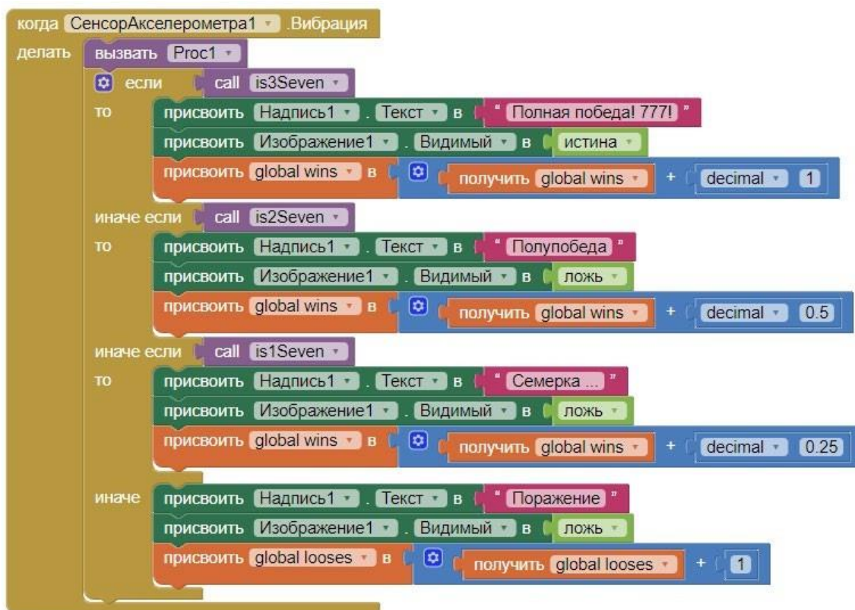
Рисунок 197. Программные блоки, выполняемые при встряхивании мобильного устройства
