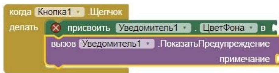
Рисунок 94. Промежуточный вид блоков обработчика
