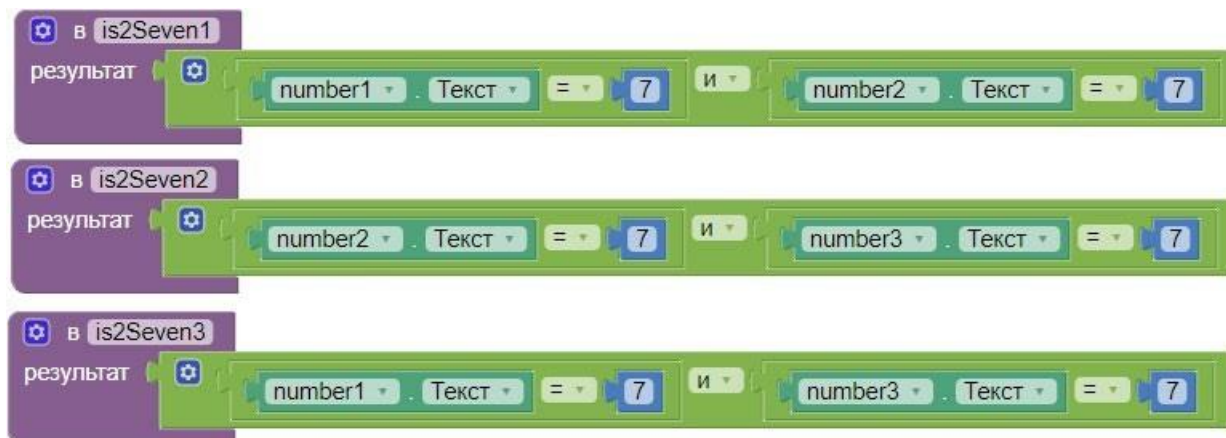
Рисунок 192. Процедуры is2Seven1, is2Seven2, is2Seven3
