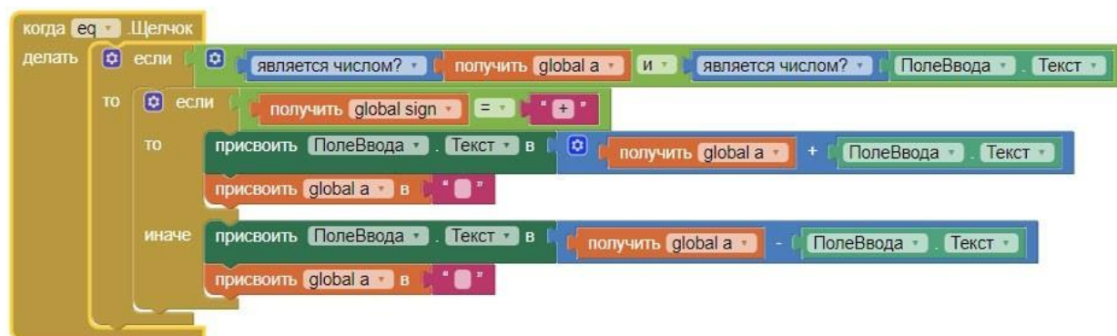
Рисунок 154. Схема блоков для кнопки «=»
