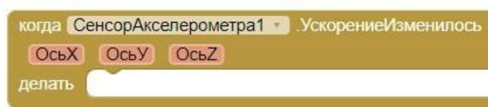
Рисунок 292. Обработчик события изменения ускорений мобильного устройства по координатным осям
