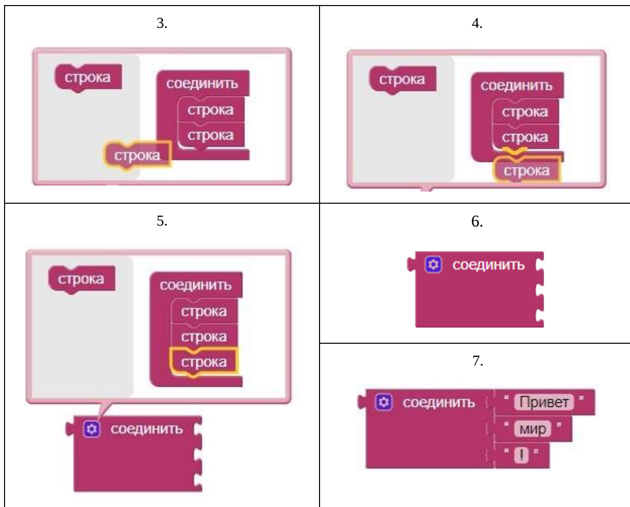
Рисунок 74. Последовательность работы с мутатором блока «соединить»
