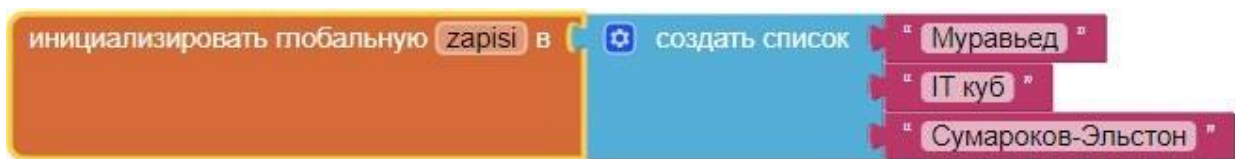
Рисунок 222. Инициализация массива
