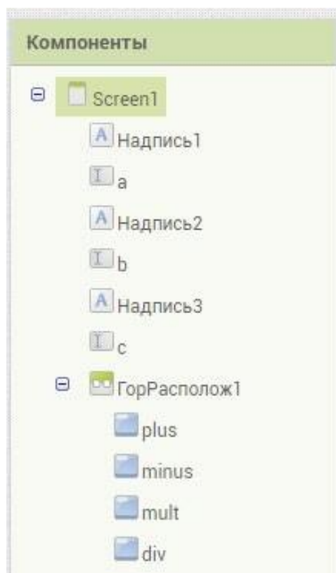
Рисунок 121. Схема компонент
