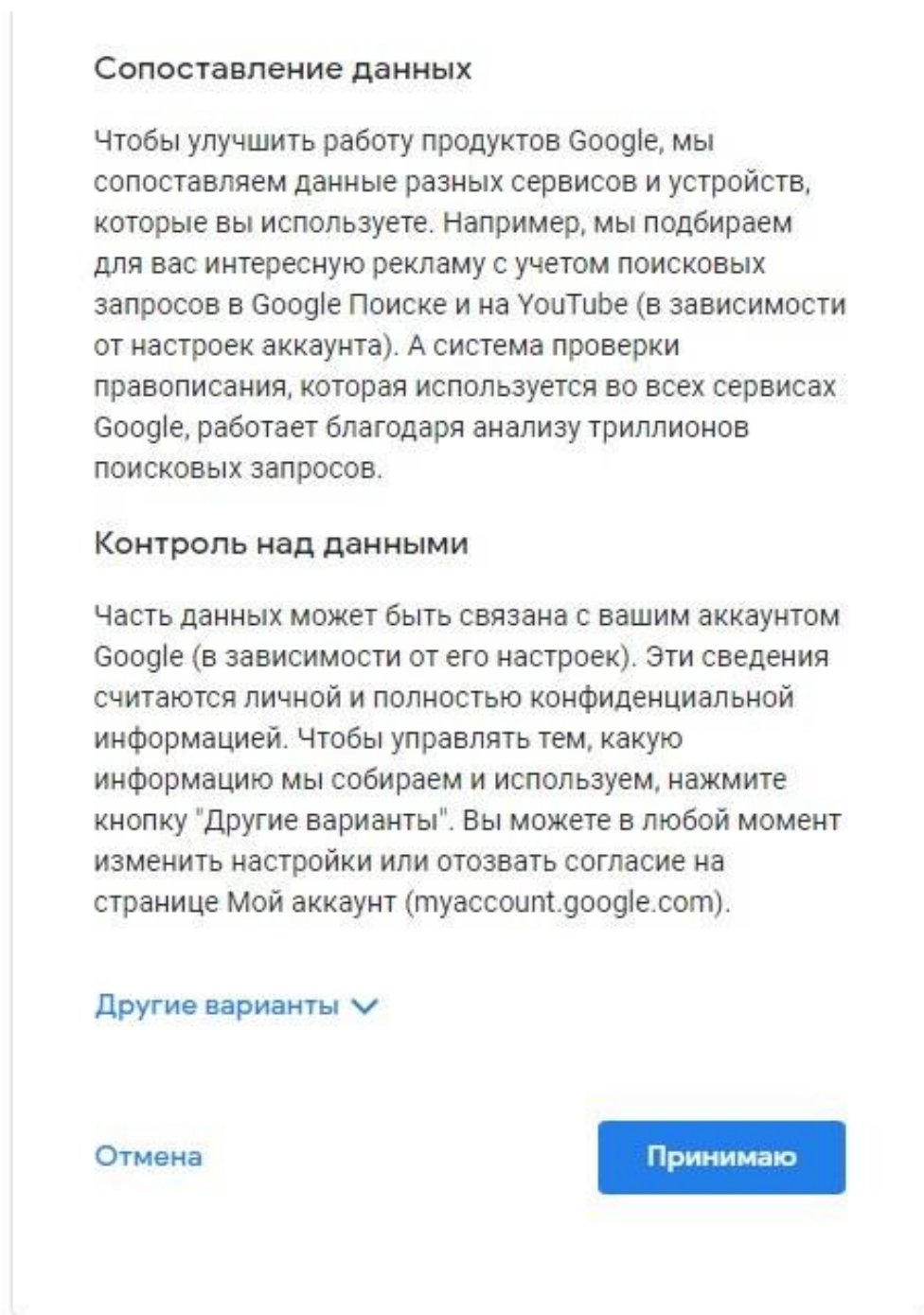
Рисунок 12. Подтверждение договора
