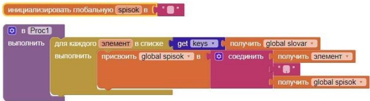
Рисунок 263. Процедура заполнения массива spisok значениями ключей словаря
