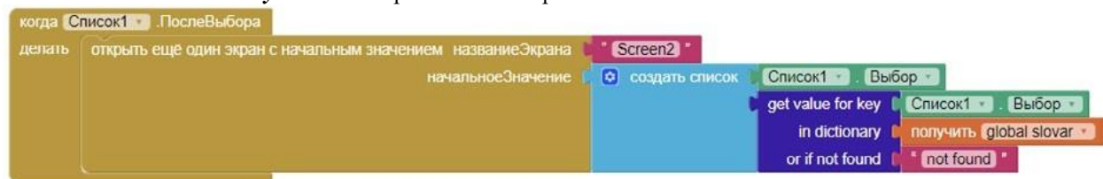
Рисунок 265. Обработчик выбора элемента компоненты Список1
