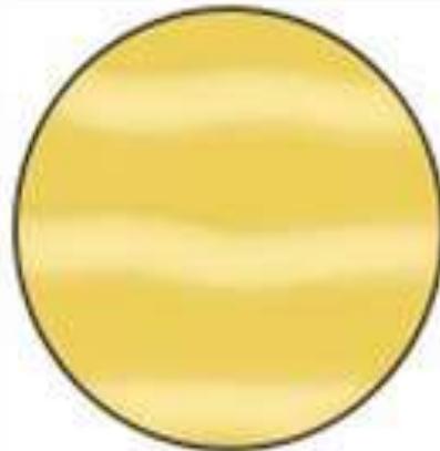
Венера
