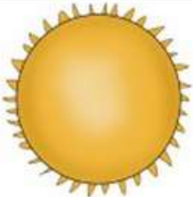
Солнце
