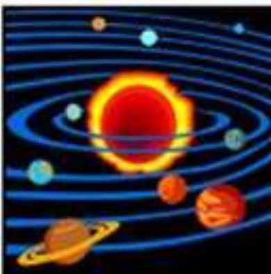
солнечная система
