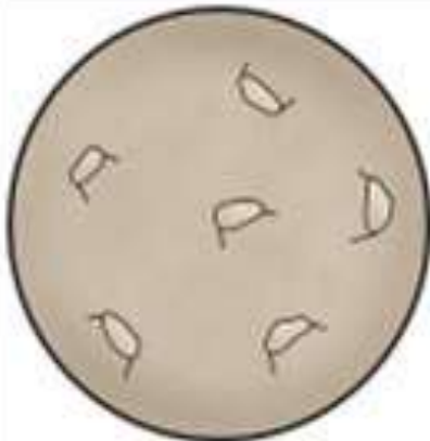
Меркурий
